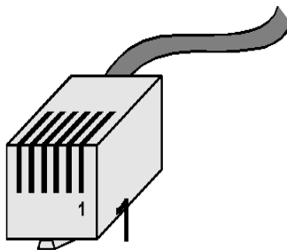
6pol RJ für TBT-Geräte
