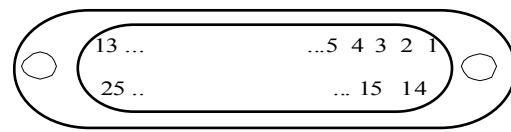
Lötseite von hinten
