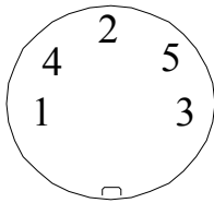
5p DIN Stecker von hinten
